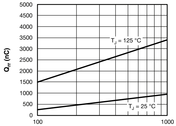
93635_08 di F /dt (A/μs)
