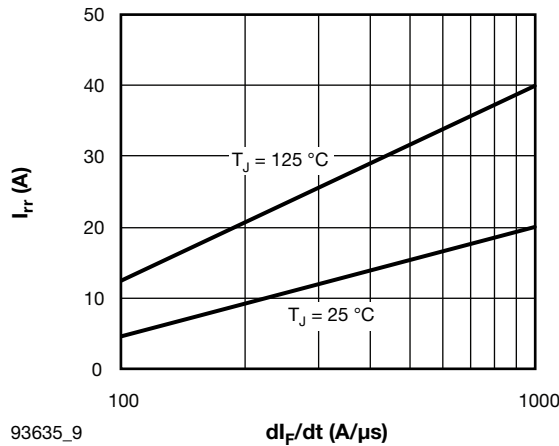
Fig. 9 - Typical I rr Diode vs. di F /dt
