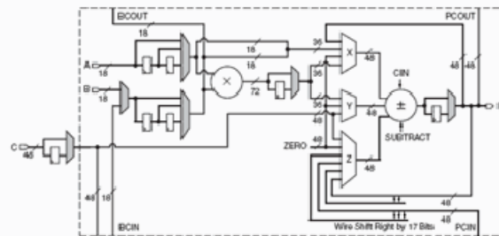
Virtex4 DSP48 Math Slice
