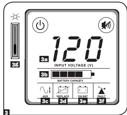
Pantalla LCD
